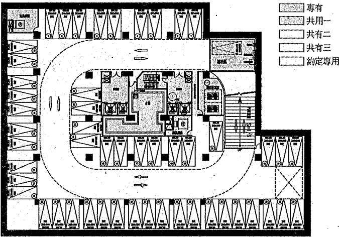
地下四層平面圖 A13-B1/200
