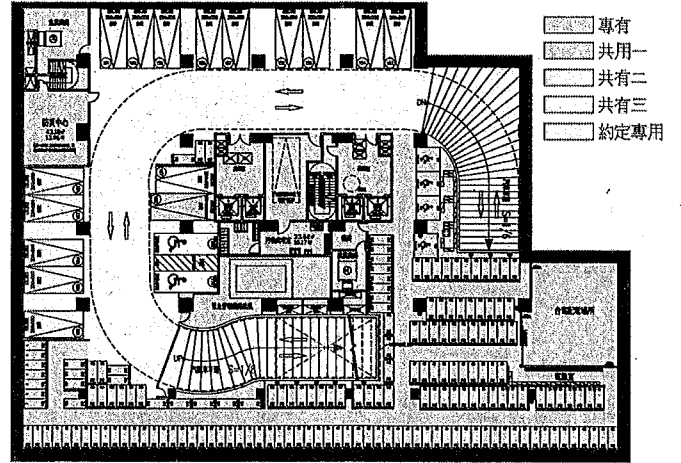
地下一層平面圖 A13-B1/200
