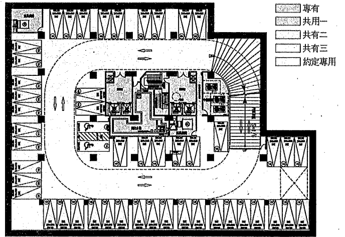
地下二層平面圖 A13-B1/200
