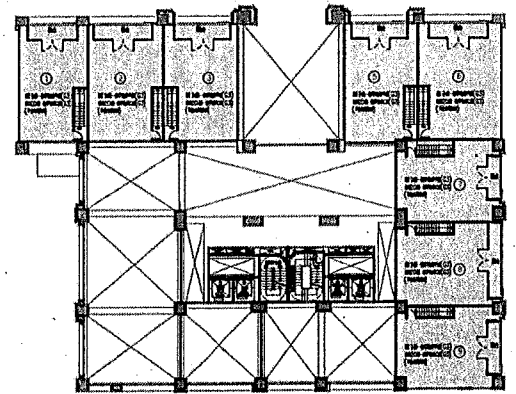
十三樓平面圖 設計師
