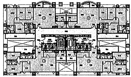
■ 十四層平面圖 1/1000
