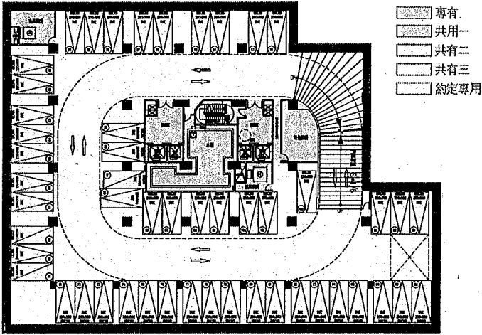
地下三層平面圖 A13-B1/200
