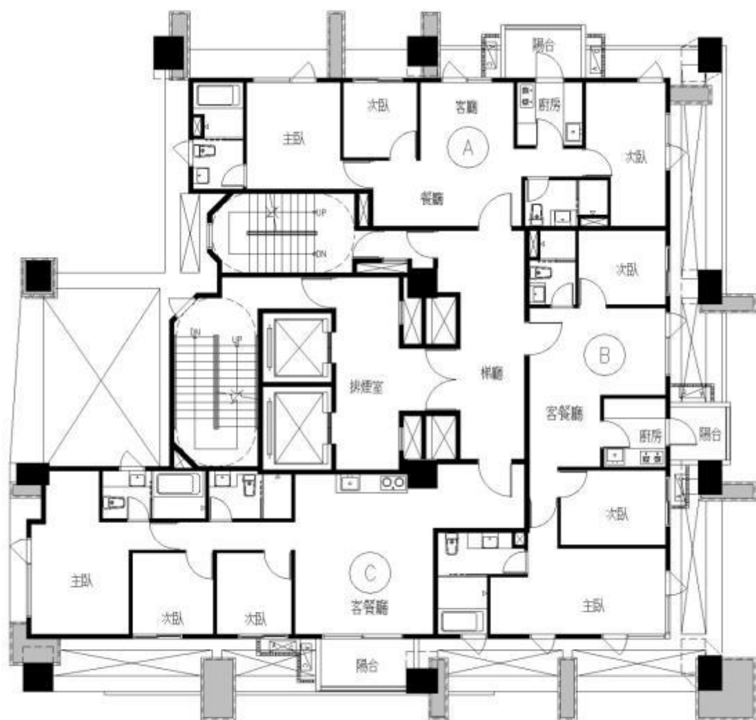
十九層平面圖
