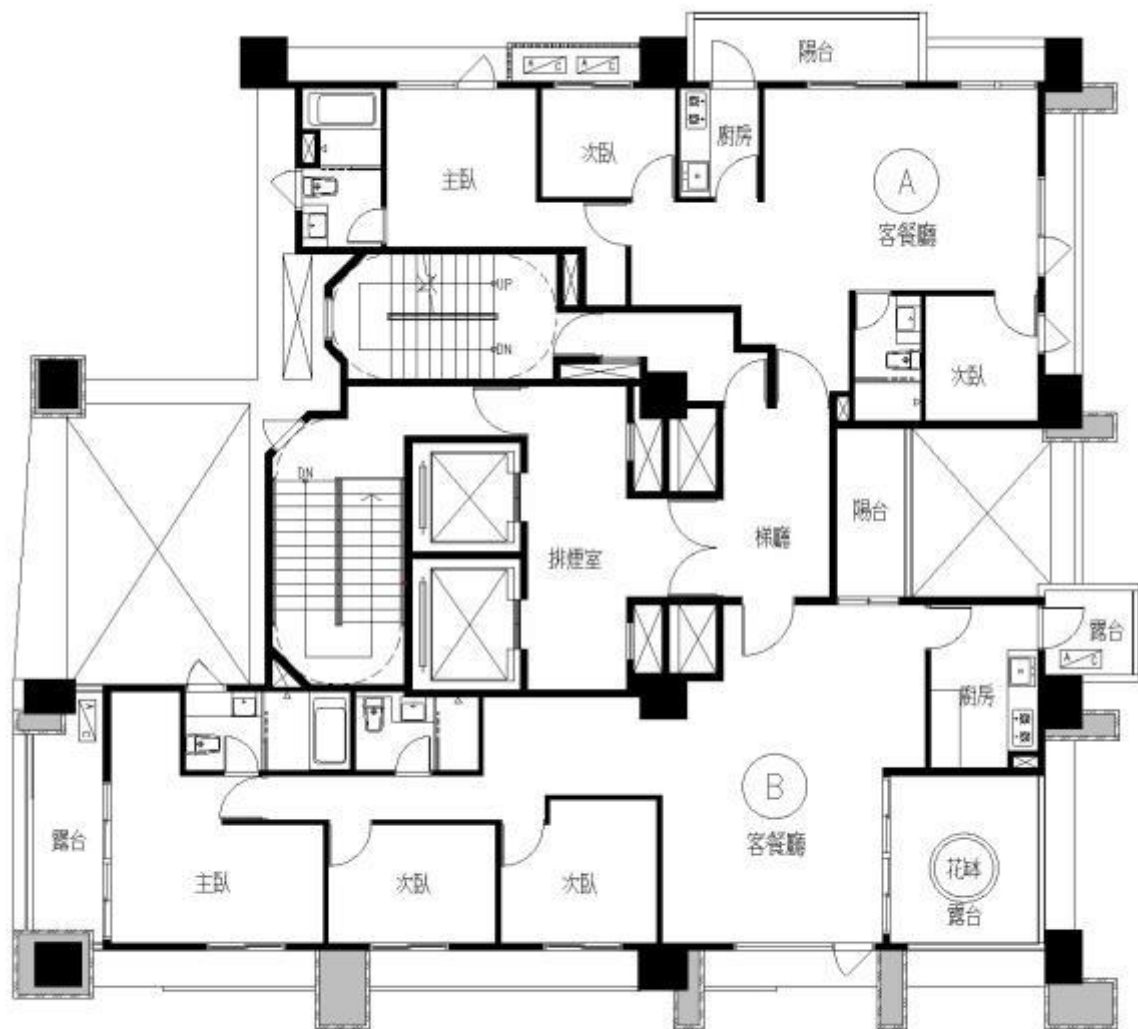
二十一層平面圖
