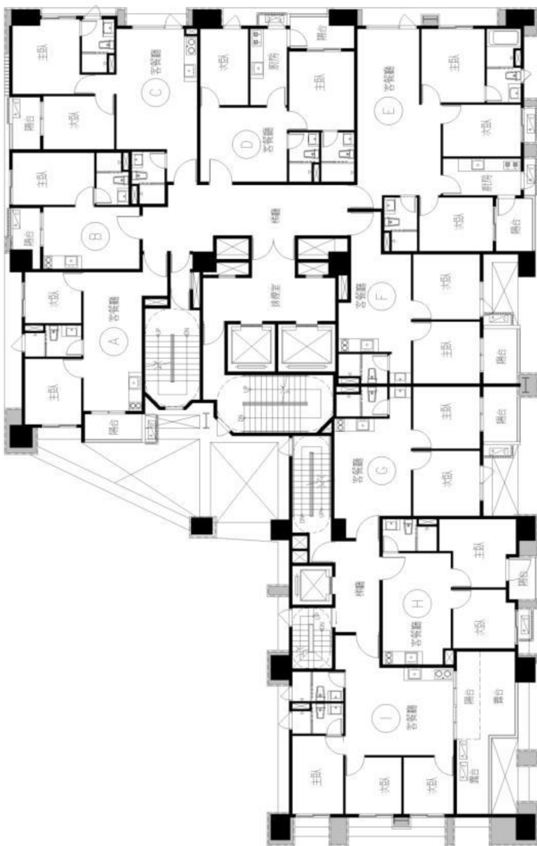
九層平面圖
