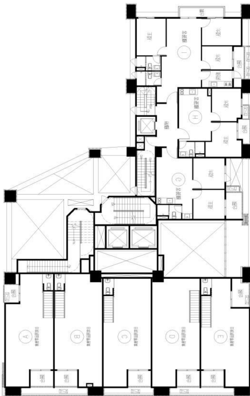
圖面平圖二
