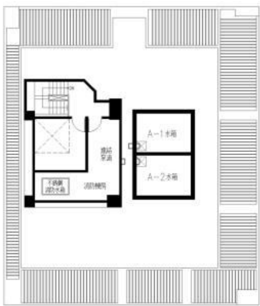
屋突三層平面圖
