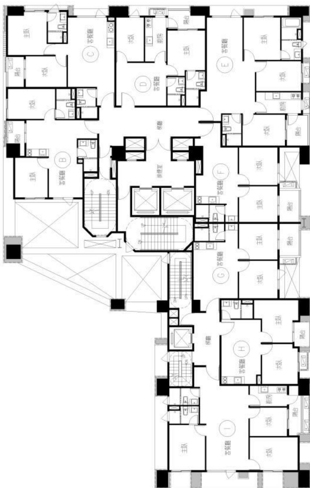
三層平面圖
