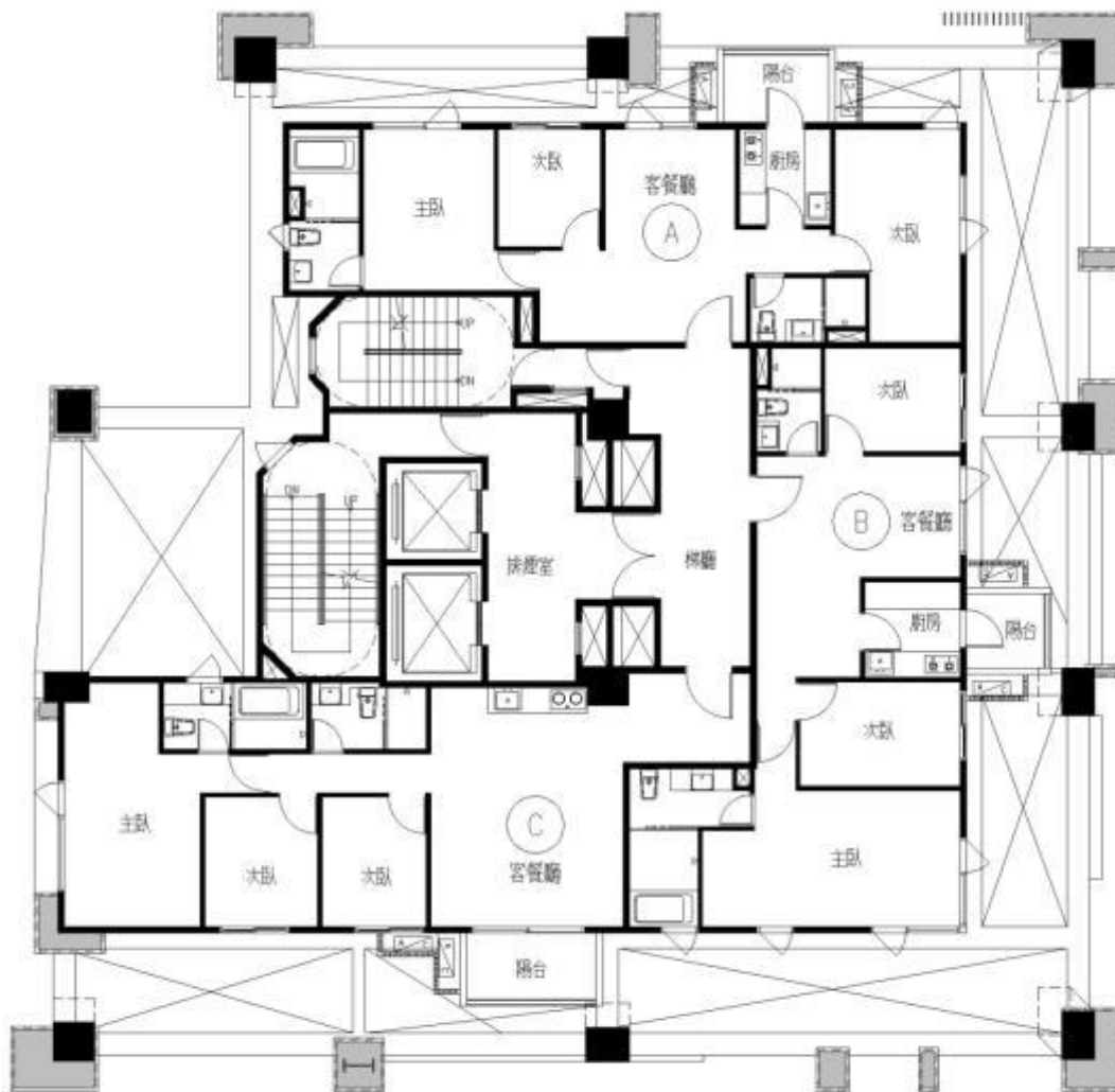
十六層平面圖
