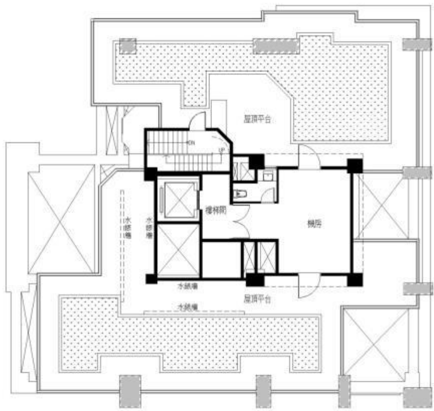
屋突一層平面圖
