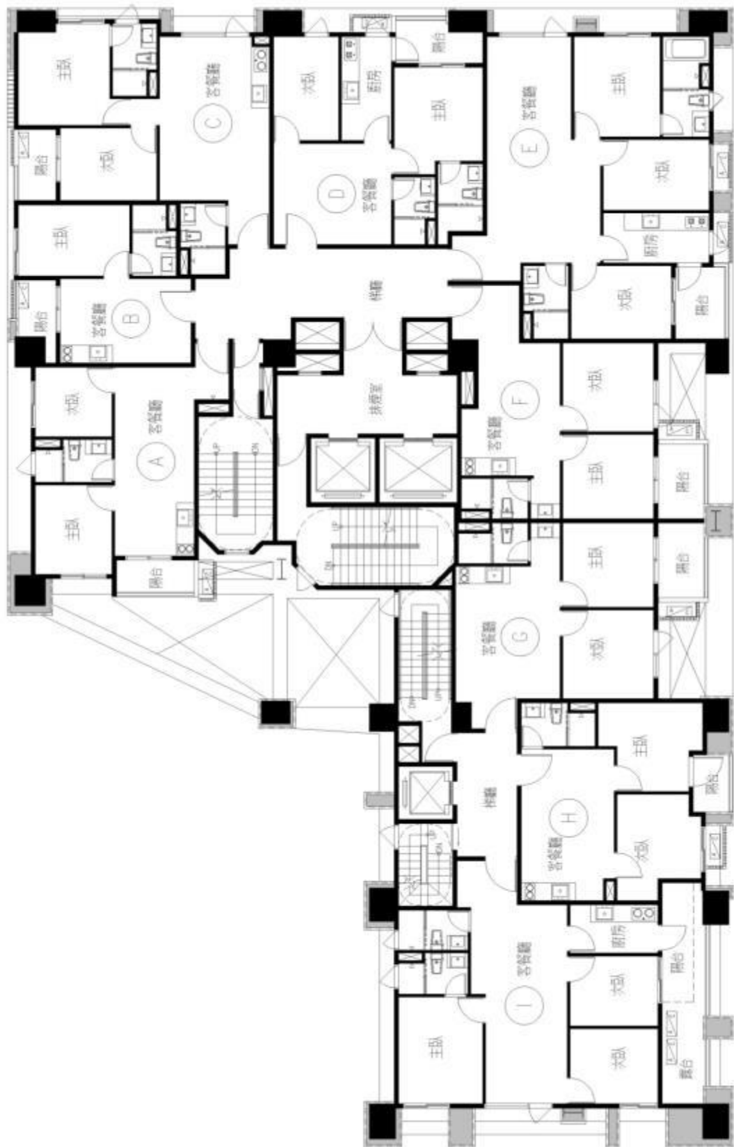
七層平面圖
