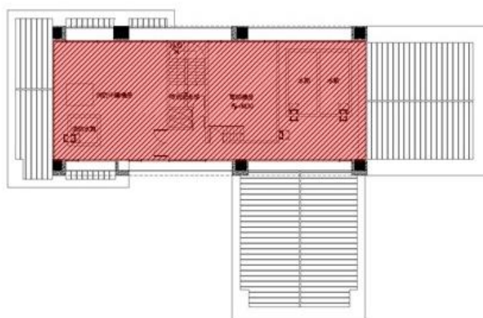
屋突二層平面圖
