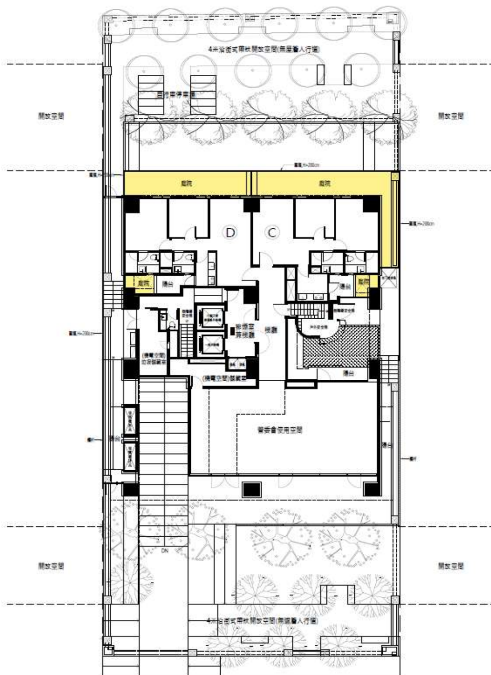
一層平面圖
