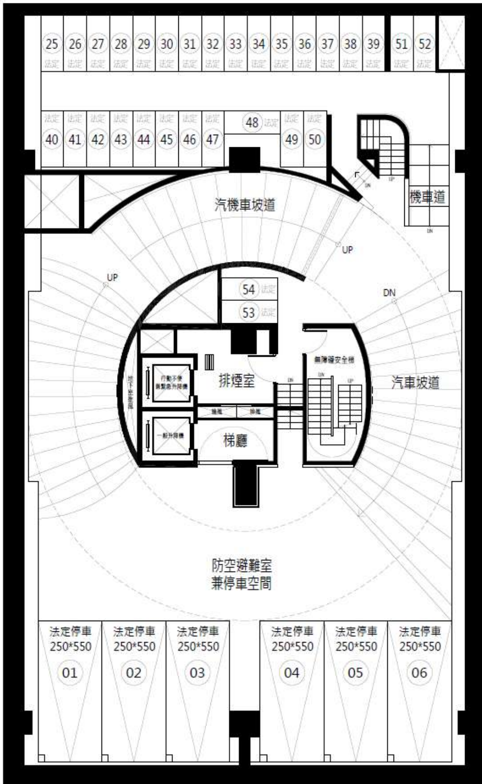
N ▲ 地下二層平面圖
