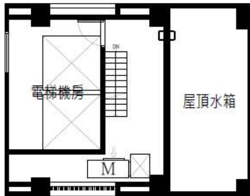
屋突三層平面圖
