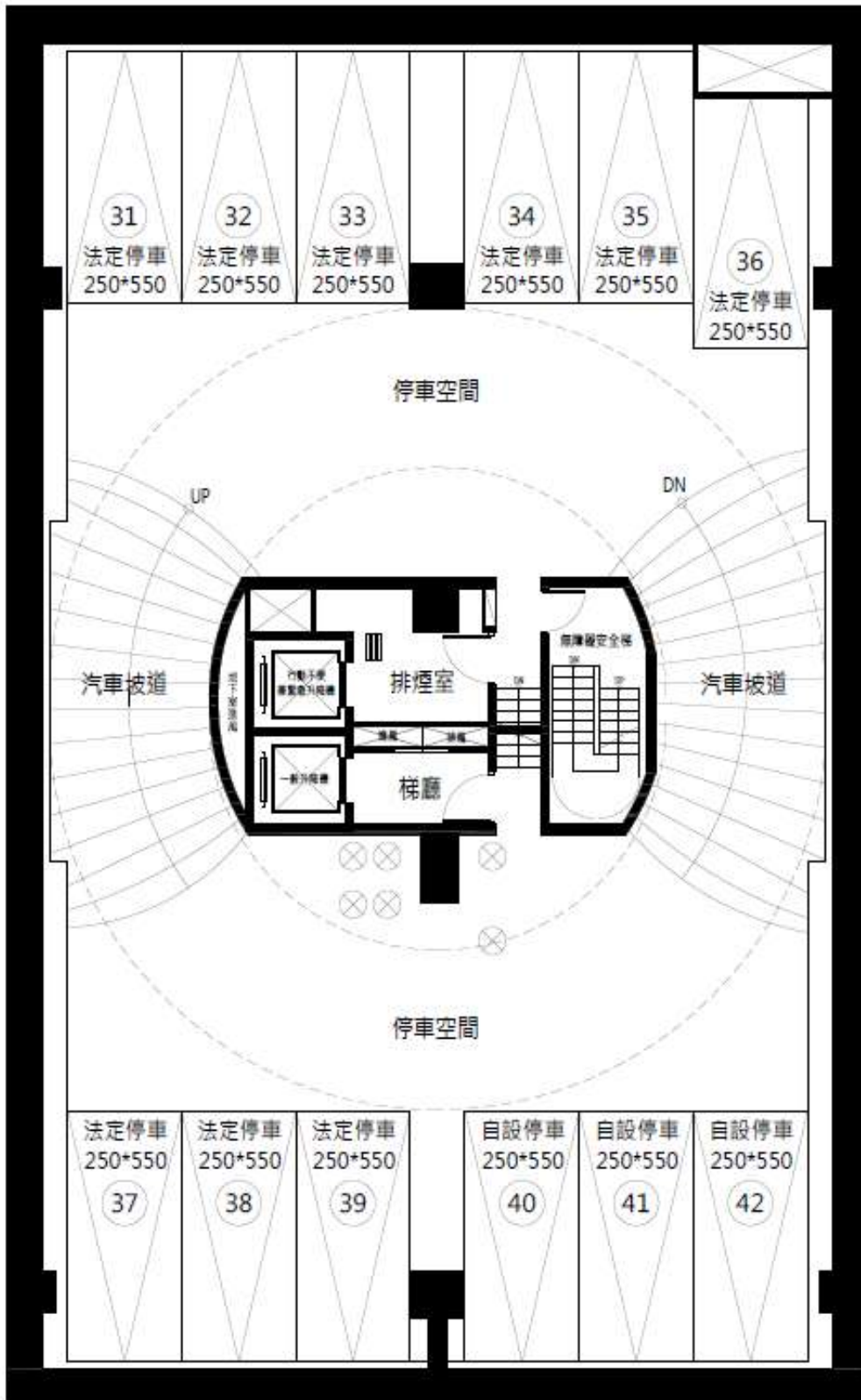
Ⓝ 地下五層平面圖
