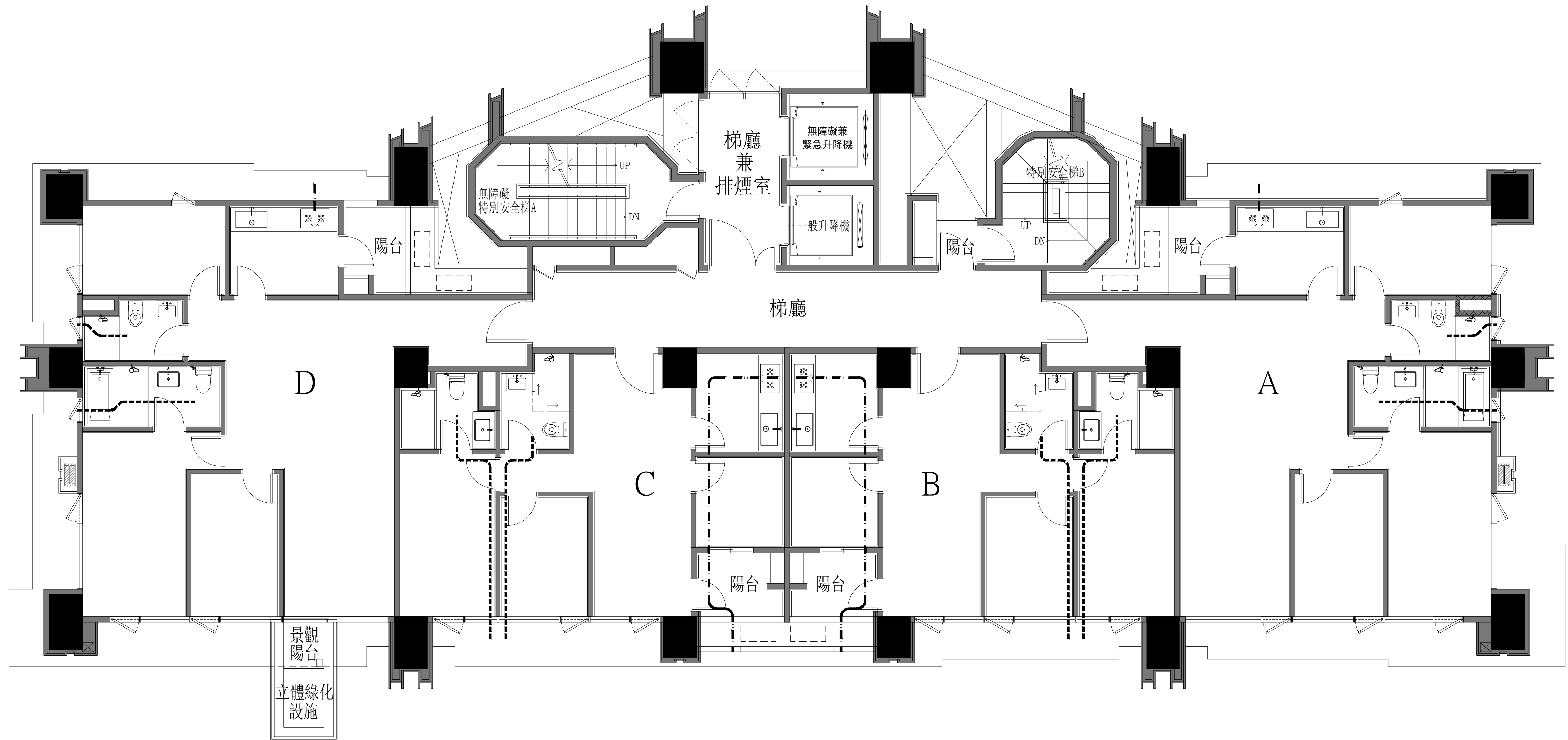
十一層平面圖
