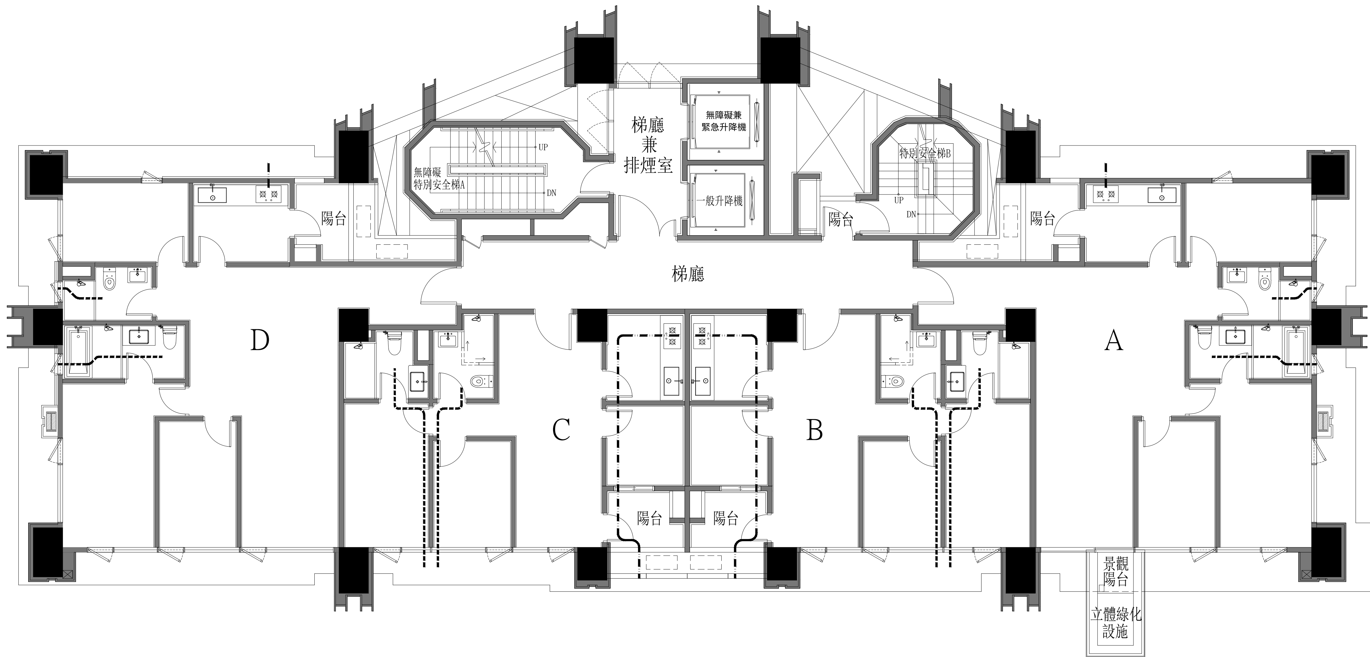
十四層平面圖
