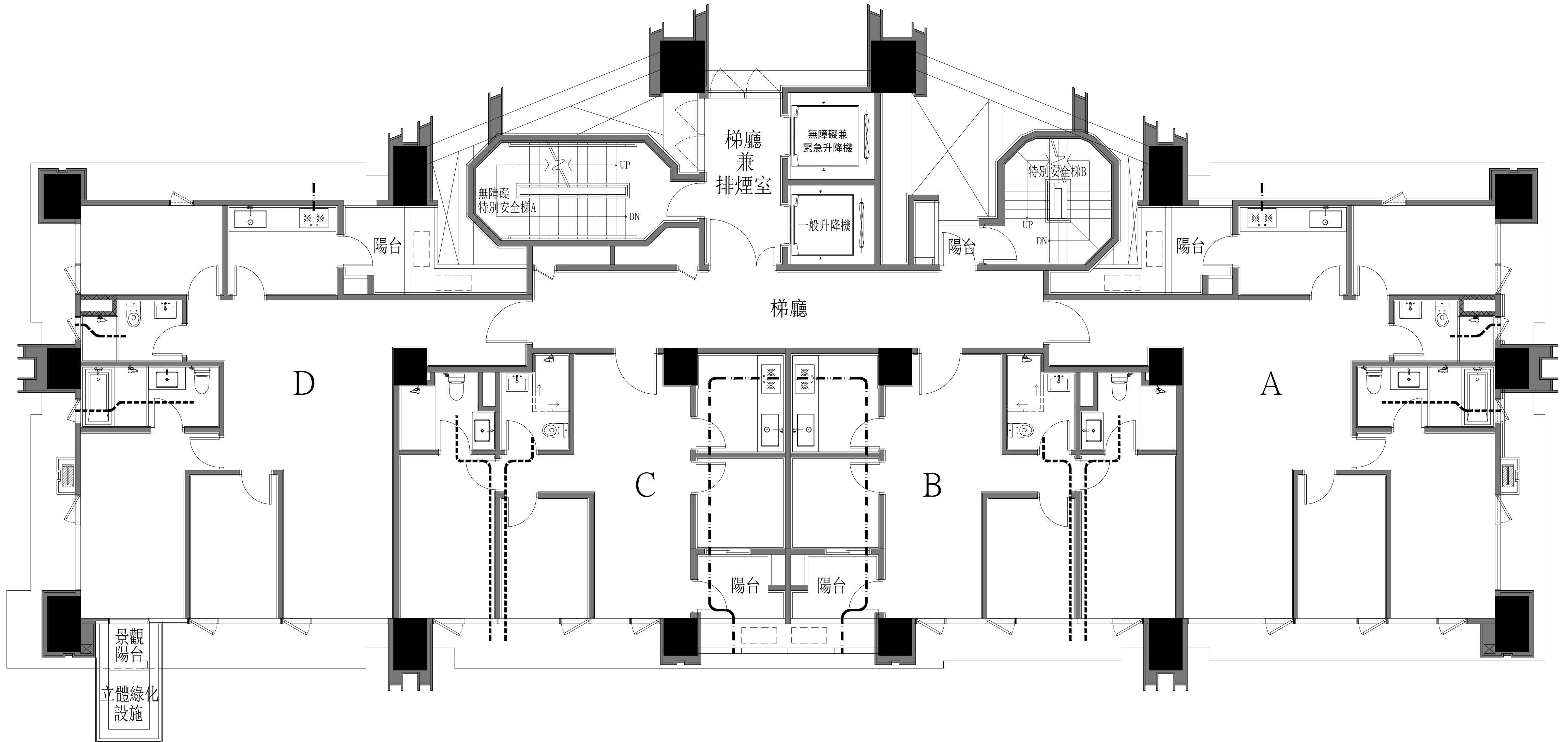
十三、十八層平面圖
